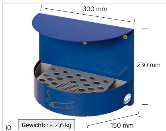
Abb.: Wandascher H 23 blau (28702)
