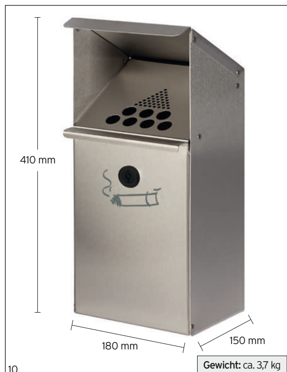
Abb.: Wandascher WH 41, Art.-Nr. 1205
