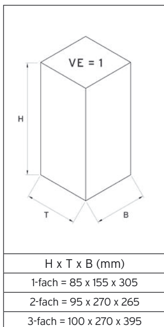
Abb.: Art.-Nr. 5931, Wandspender, 2-fach
