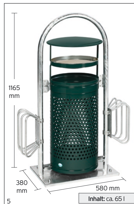
Abb.: Rohrbogenständer RB 001, Art.-Nr. 1862
