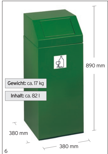
Abb.: Wertstoffsammler 76 L Grün-Glas, Art.-Nr. 1242
