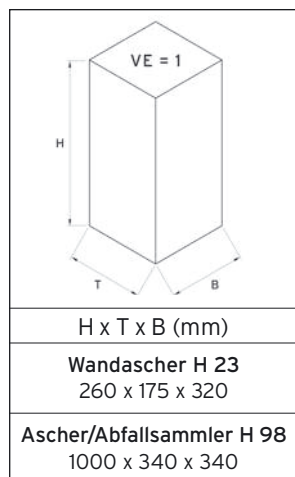
Abb.: Wandascher H 23 blau (28702)
