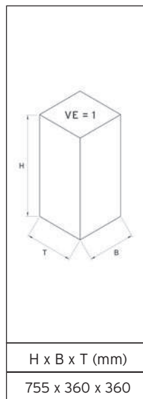
Abb.: Art.-Nr. 21307 Optional mit Rollensatz Art.-Nr. 3669
