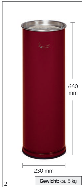
Abb.: Ascher H 66 purpurrot beschichtet, Art.-Nr. 17131
