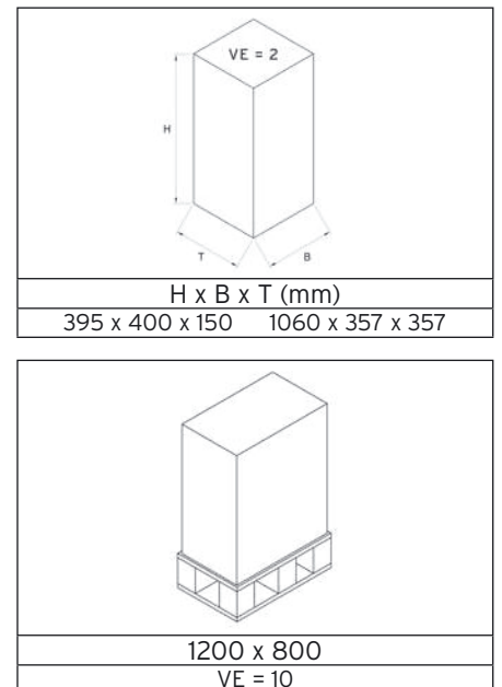
Abb.: Artikel-Nr. 2016 + 2017 (Station in Edelstahl fahrbar)
