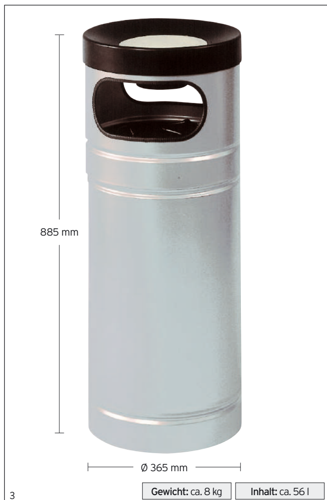
Abb.: Abfallsammler / Ascher H90, silber besch., Art-Nr.: 1116
