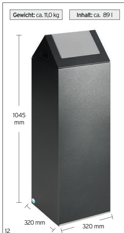
Abb.: WSG 85S, antik-silber, Einwurfklappe silber, Art.-Nr. 21132
