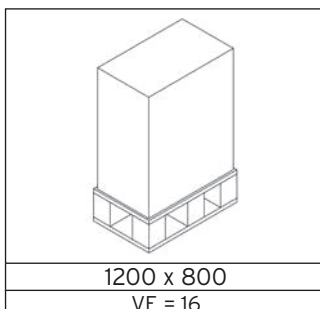
Abb.: Maße Spender (Artikel 2080 - 2082)
