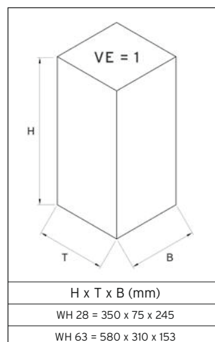
Abb.: Wandascher WH 28 Edelstahl, Art.-Nr. 45007
