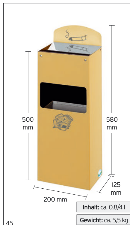
Abb.: Wandascher WH 51, Messing-Ausführung mit Schild und Aufkleber, Art.-Nr. 1962
