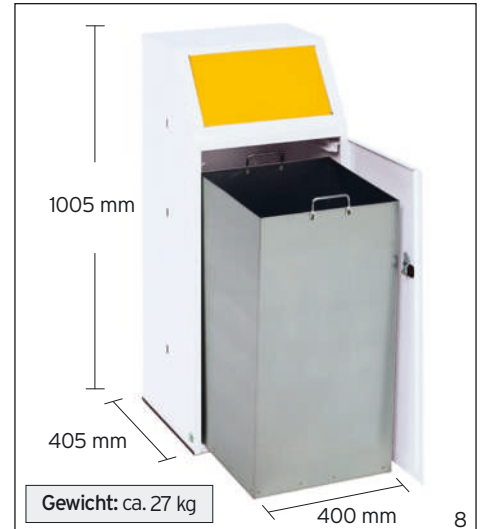
Abb.: WSG 69 mit Fronttür, Ausf. B, Einwurflappe gelb, Art.-Nr. 17161
