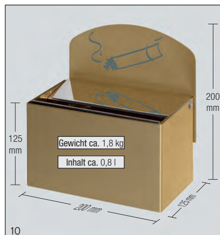
Abb.: „Wandascher“ WH 13, Messing-Ausführung mit Schild und Aufkleber Art.-Nr. 1961
