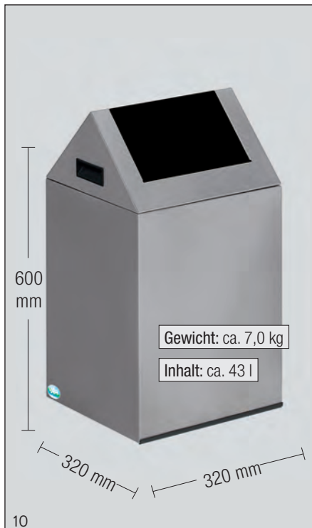
Abb.: WSG 40S, silber, Einwurfklappe anthrazit, Art.-Nr. 21122
