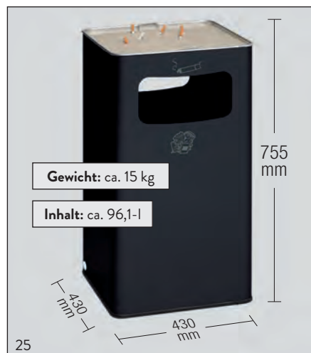
Abb.: Ascher/Abfallsammler B42 R, anthrazit, Art.-Nr. 3092
