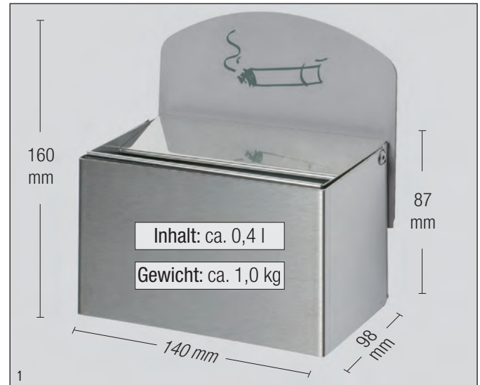
Wandascher WH 9, Edelstahl, mit Schild. Art.-Nr. 14791
