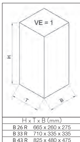
Abb.: Kombi-Ascher B 43 R Edelstahl, Art.-Nr. 3479
