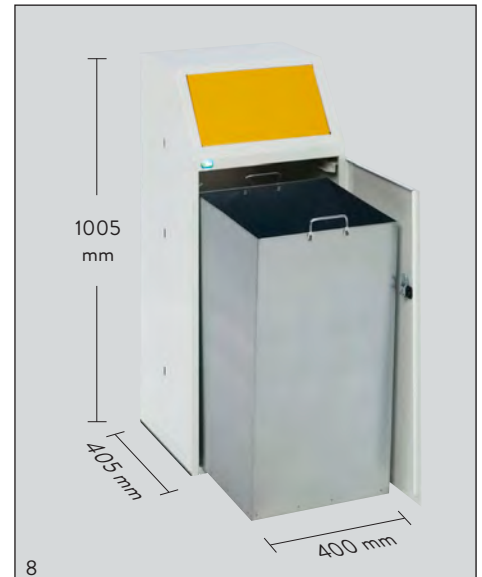
Abb.: WSG 69 mit Fronttür, Ausf. B, Einwurflappe gelb, Art.-Nr. 17161
