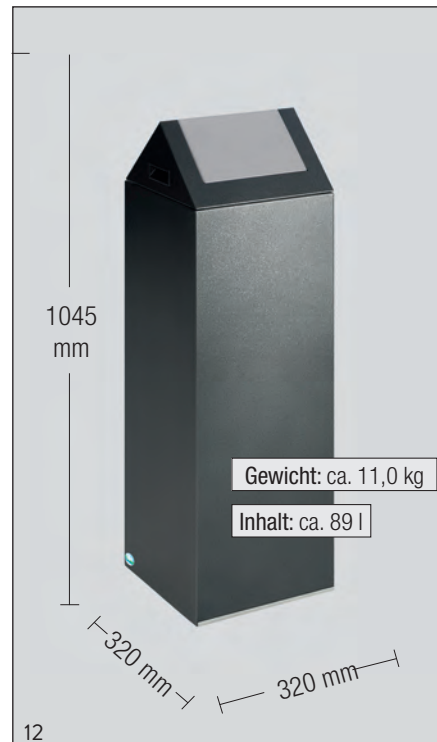
Abb.: WSG 85S, antik-silber, Einwurfklappe silber, Art.-Nr. 21132
