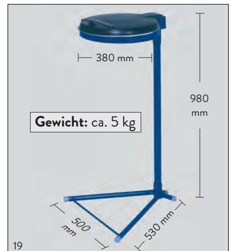
Abb.: Modell „Standard, enzianblau besch.“ mit KS-Deckel, Art.-Nr. 10203
