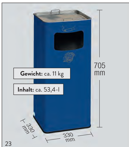
Abb.: Ascher/Abfallsammler B32 R, enzyanblau, Art.-Nr. 3083
