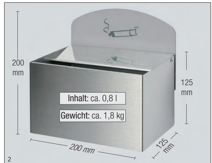
Wandascher WH 13, Edelstahl, mit Schild. Art.-Nr. 14891
