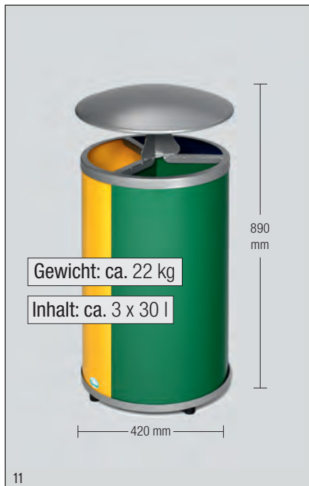
Abb.: Wertstoffstation mit Dach. Art.-Nr. 3663
