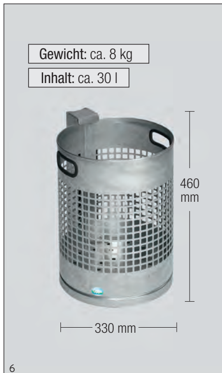
Abb.: Abfallsammler Typ WR 3, Art.-Nr. 1182
