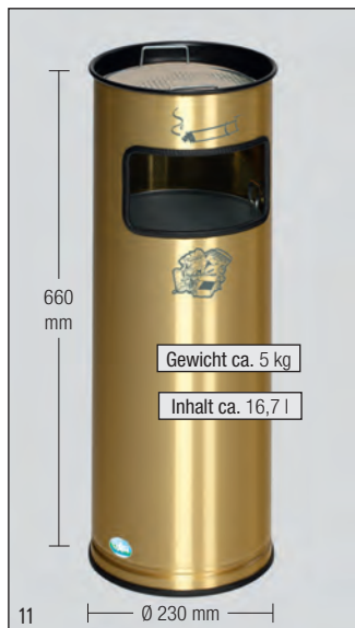
Abb.: Abfallsammler/Ascher H 66 Messing/Stahl-Ausführung Art.-Nr. 1190
