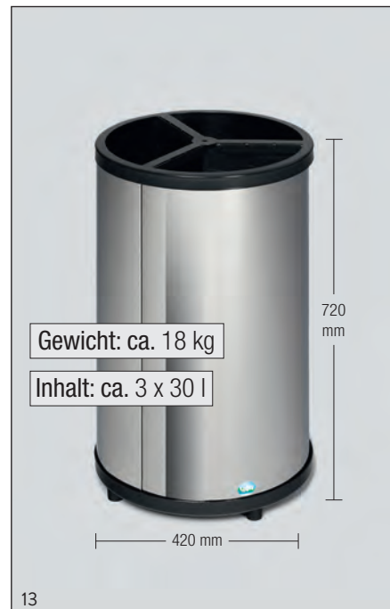
Abb.: Wertstoffstation, VA-Ausführung. Art.-Nr. 3666
