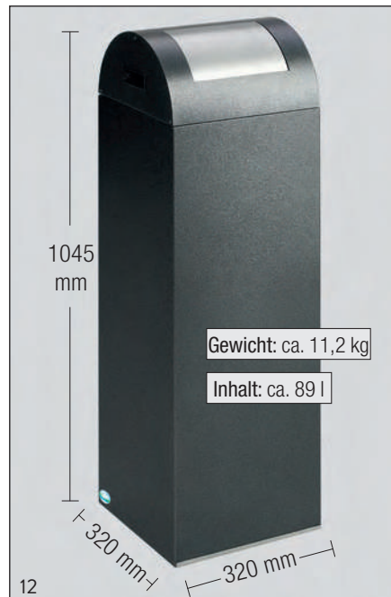
Abb.: WSG 85R, antik-silber, Einwurflappte silber, Art.-Nr. 21092
