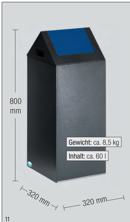
Abb.: WSG 55S, antik-silber, Einwurfklappe enzianblau, Art.-Nr. 21021
