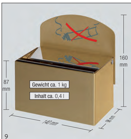
Abb.: „Wandascher“ WH 9, Messing-Ausführung mit Schild und Aufkleber Art.-Nr. 1960
