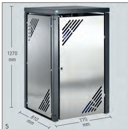
Abb.: Müllbehälterschrank MBS 2, Art.-Nr. 21251
