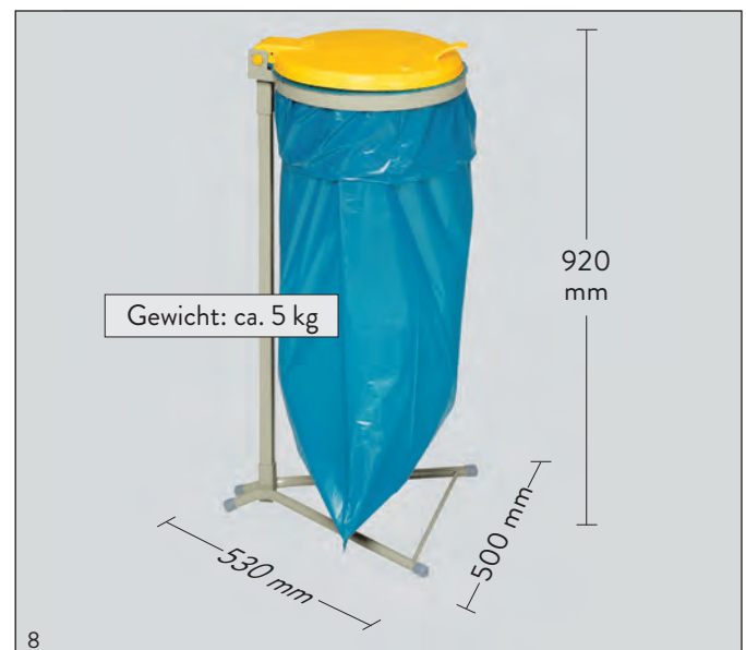
Abb.: Abfallsammler WS 120, Deckel gelb, Lieferung zerlegt. Einfache Selbstmontage. Art.-Nr.: 1680
