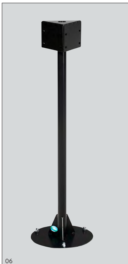
Foto 06: Standrohrbefestigung dreifach, RAL 7021, Artikel Nr. 19402
