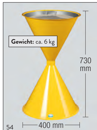
54 Ausführung gelb, mit Einlege- teil und verzinktem Sieb. Art.-Nr. 1169
