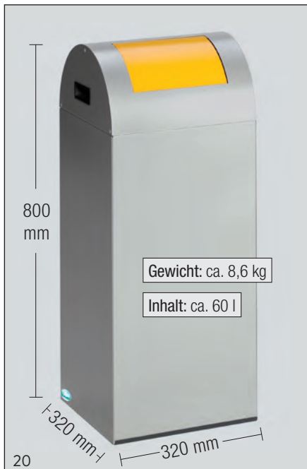
Abb.: WSG 55R, silber, Einwurflappte gelb, Art.-Nr. 21010
